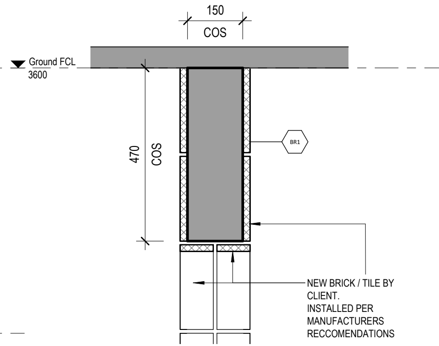
1 HEADER SECTION 1 : 10
