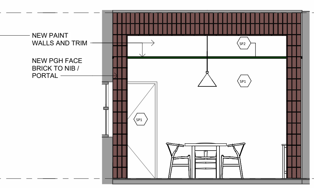
3 FUNCTION ROOM ELE 03 1 : 50
