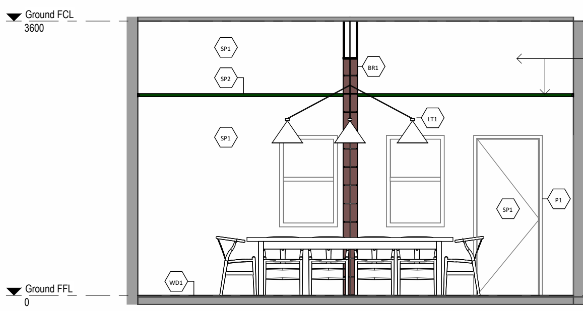
2 FUNCTION ELEVATION 02 1 : 50
